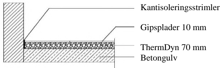
Fig. 4: Tværsnit af prøven
